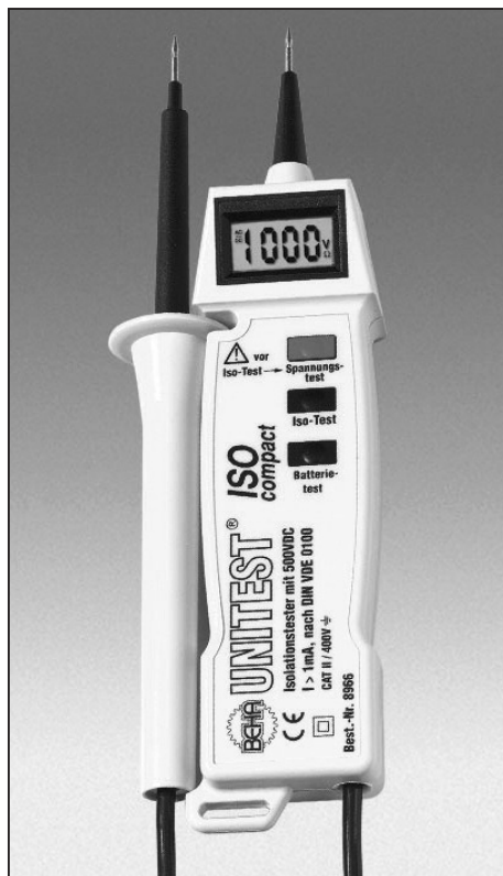
Měřič izolace Unitest ISO-COMPACT
