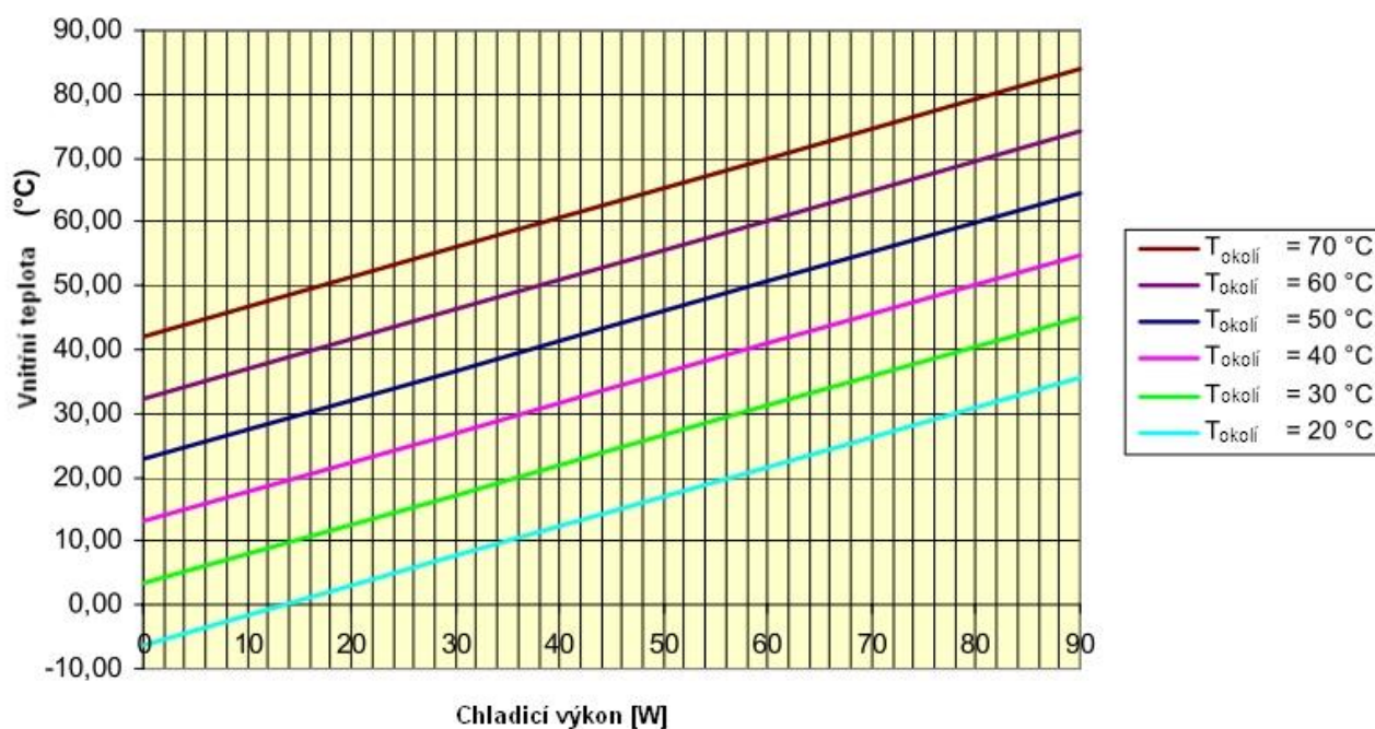
Graf chladicího výkonu FN-104-C
