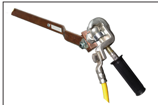
Erdung an Kugelfestpunkt
