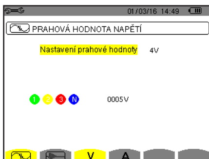
Obrázek 28: Obrazovka prahových hodnot proudu v nabídce pro režim přechodových jevů
