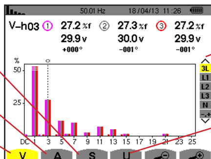
Obrázek 51: Obrázovka režimu harmonických
