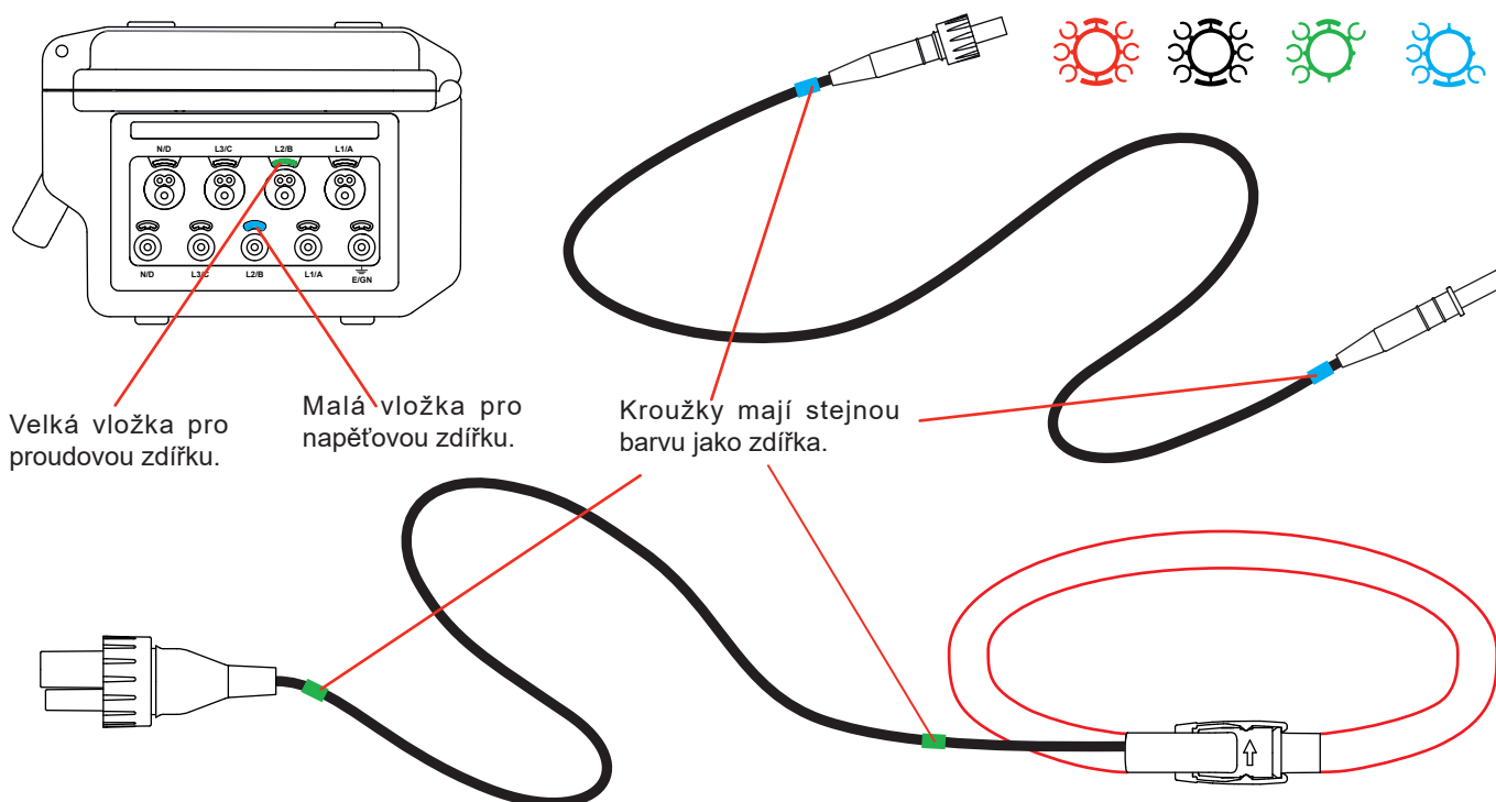
Obrázek 8: značení kabelů
