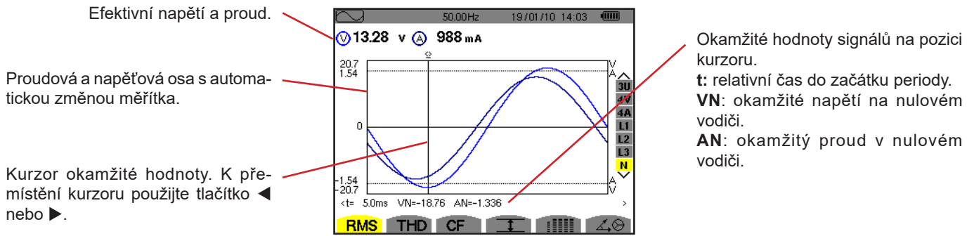
Obrázek 66: Obrazovka RMS pro nulový vodič
