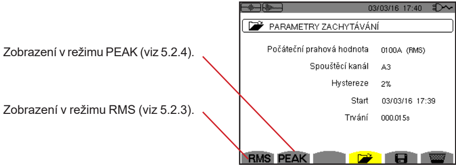
Obrázek 43: Obrazovka parametrů zachycení
