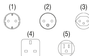
Jednotlivá provedení zásuvek
