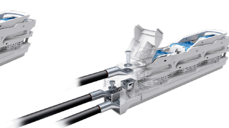
Šroubové připojení M8
