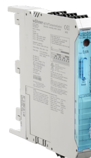
Provedení na 30 mm systém
