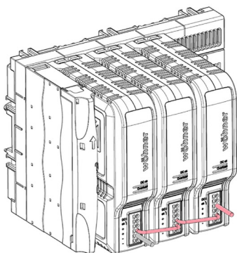
Příklad sériového propojení zvyšující výstupní napětí
