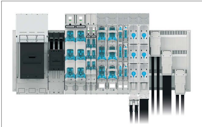
Obr. 1. Systém přípojníc 185 Power
