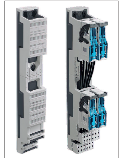
Obr. 3. Adaptér EQUES se systémem CrossBoard
